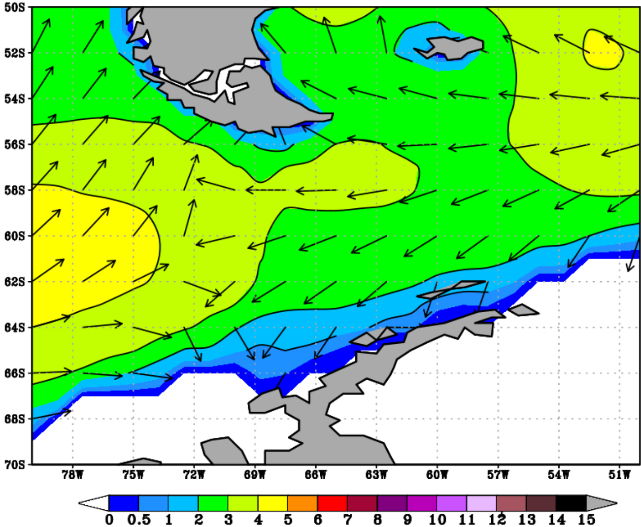
ALTURA DE OLA SIGNIFICATIVA, EN METROS Datos grib Modelo Global NWW3 corrida 06Z12JUL2020 res 0.5°x0.5° procesado con GrADS
